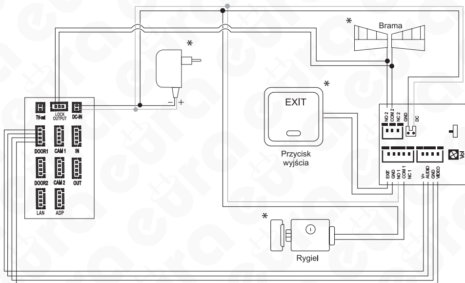
Rys. 5. Schemat podłączenia z wykorzystaniem jednego zasilacza (12V 4,5A z funkcją regulacji napięcia)
