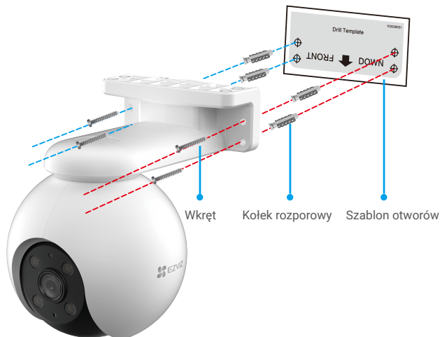
Rys. 2 Montaż ścienny
