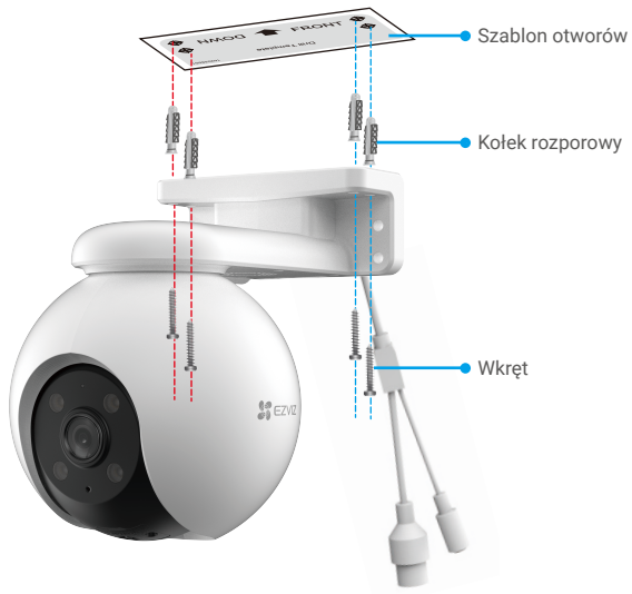
Rys. 1 Montaż sufitowy
