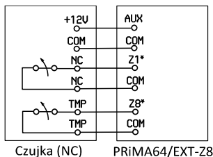
Rysunek 5: Czujka NC podłączona w konfiguracji NC
