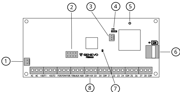
Rysunek 1: Płyta główna centrali PRiMA 64
