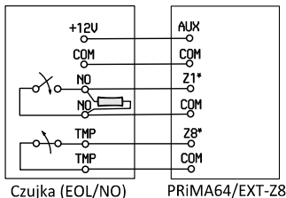
Rysunek 6: Czujka NO podłączona w konfiguracji EOL
