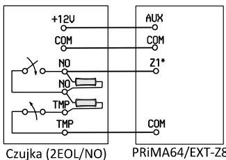
Rysunek 7: Czujka NO podłączona w konfiguracji 2EOL/NO
