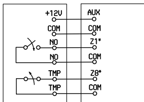
Czujka (NO) PRIMA64/EXT-Z8
