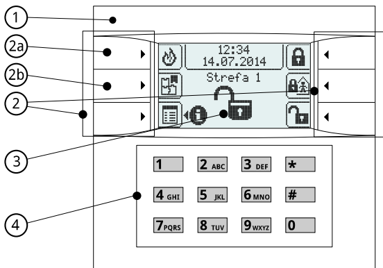
Rysunek 2: Manipulator PRiMA LCD do PRiMA 64
