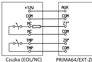
Rysunek 8: Czujka NC podłączona w konfiguracji EOL
