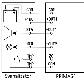
Rysunek 12: Podłączanie sygnalizatora z własnym zasilaniem
