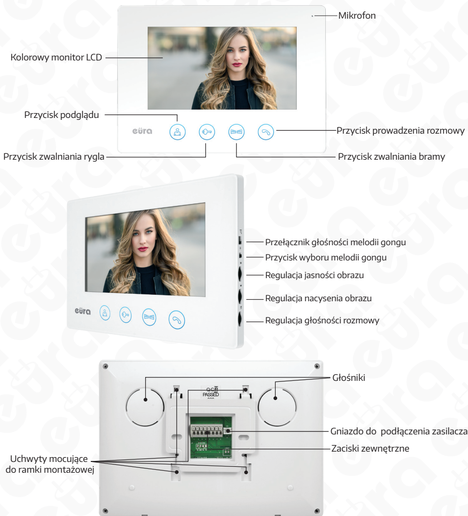
Rys. 1. Budowa monitora VDA-40A3
